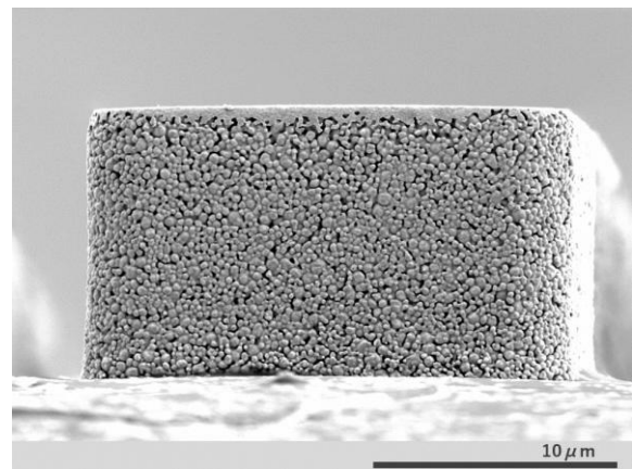
<AuRoFUSE™ Preforms 측면 SEM 이미지>
