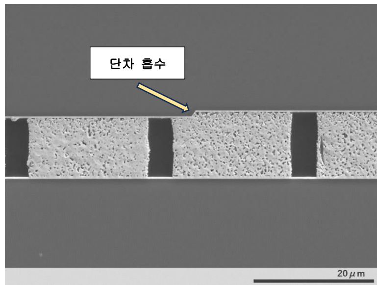
<그림 2. 접합 시 단차를 흡수하는 AuRoFUSE™ Preforms SEM 이미지>
