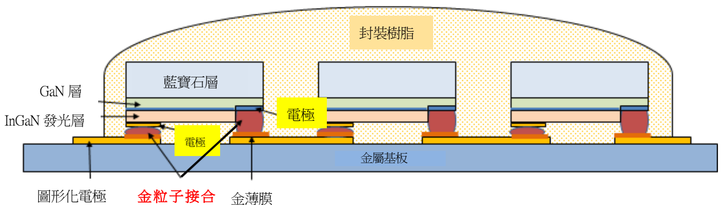
本 LED 模組之解說圖
